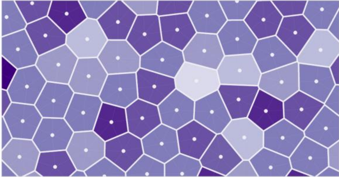
Diagramme de Voronoi
